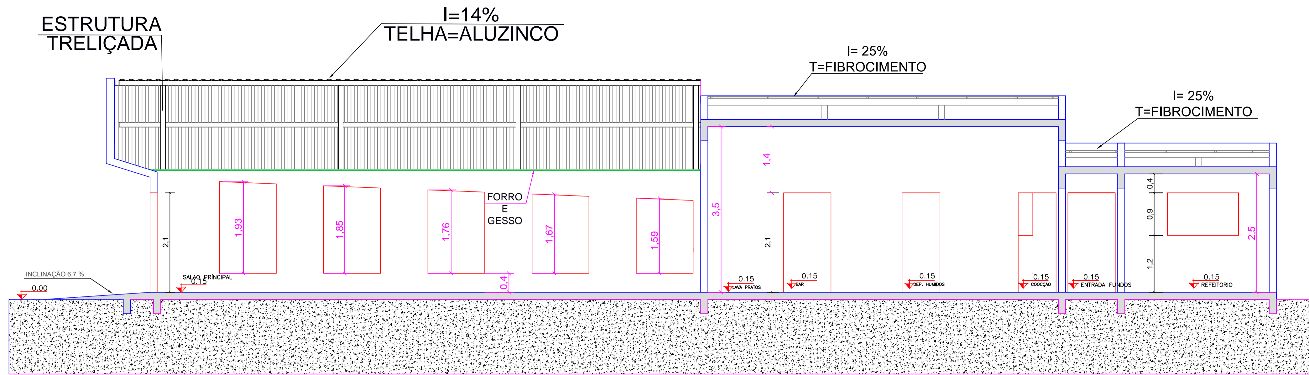
CORTE ESCALA: 1:50
