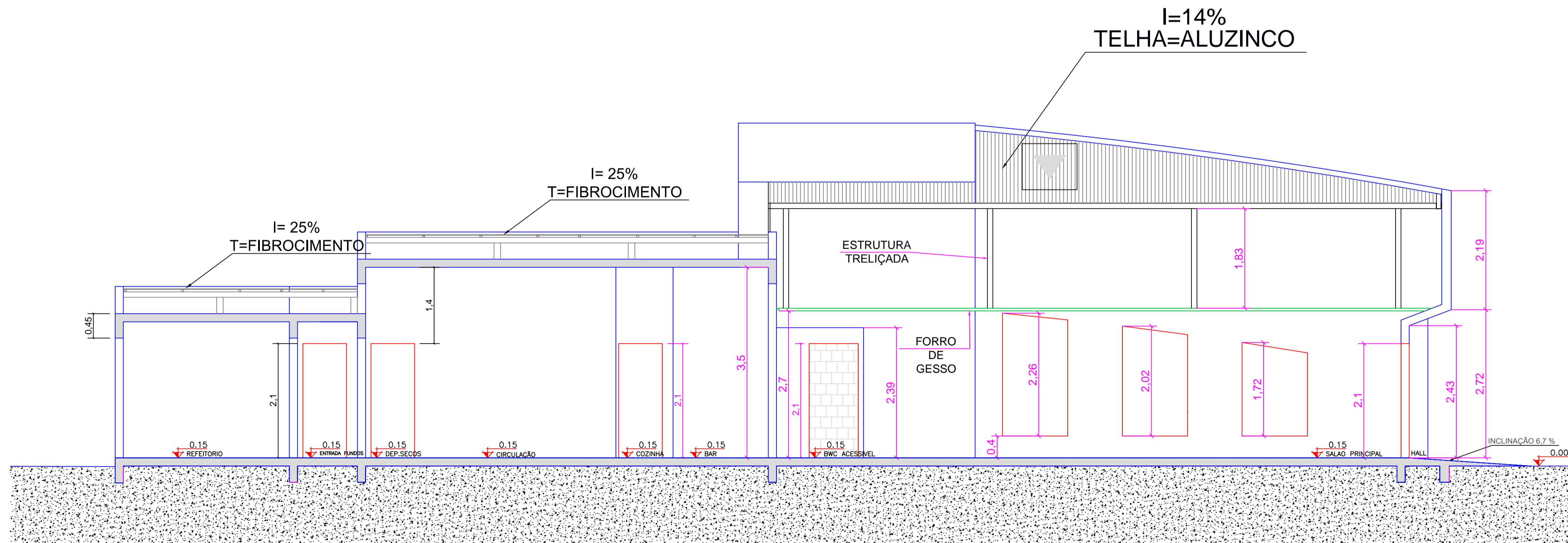
CORTE ESCALA: 1:50
